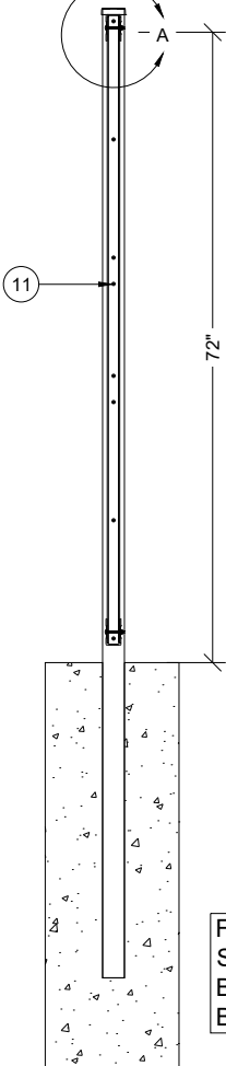
2 SECTION SCALE: 1/2" = 1'-0"
