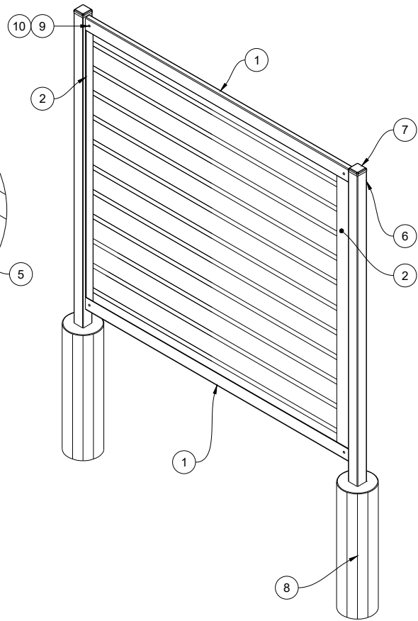
3 ISO VIEW SCALE: 1/2" = 1'-0"
